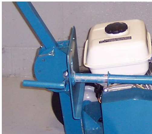
Fig. 3: Coupeuse en position de repos
